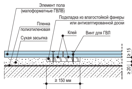
Рис. 12. Прямой стык
